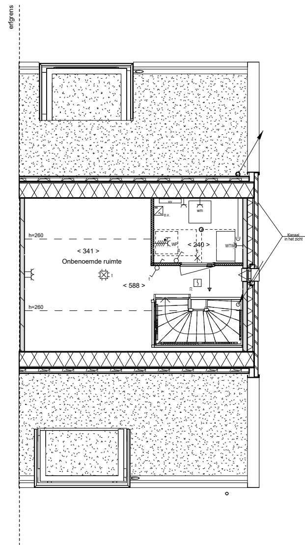
02 tweede verdieping
