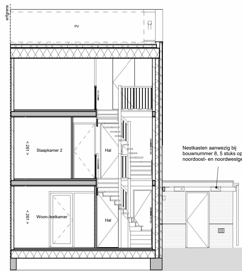
doorsnede A
