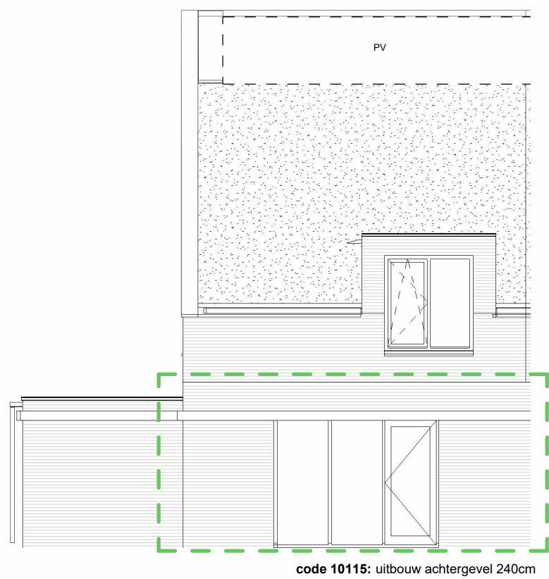
achtergevel
