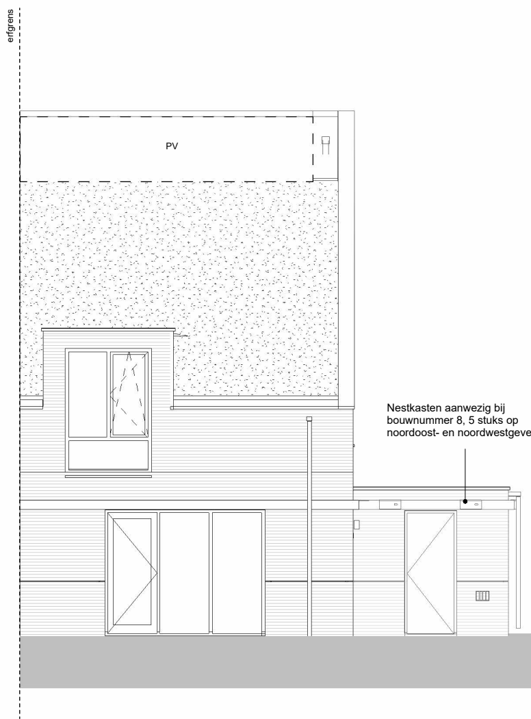
voorgevel
