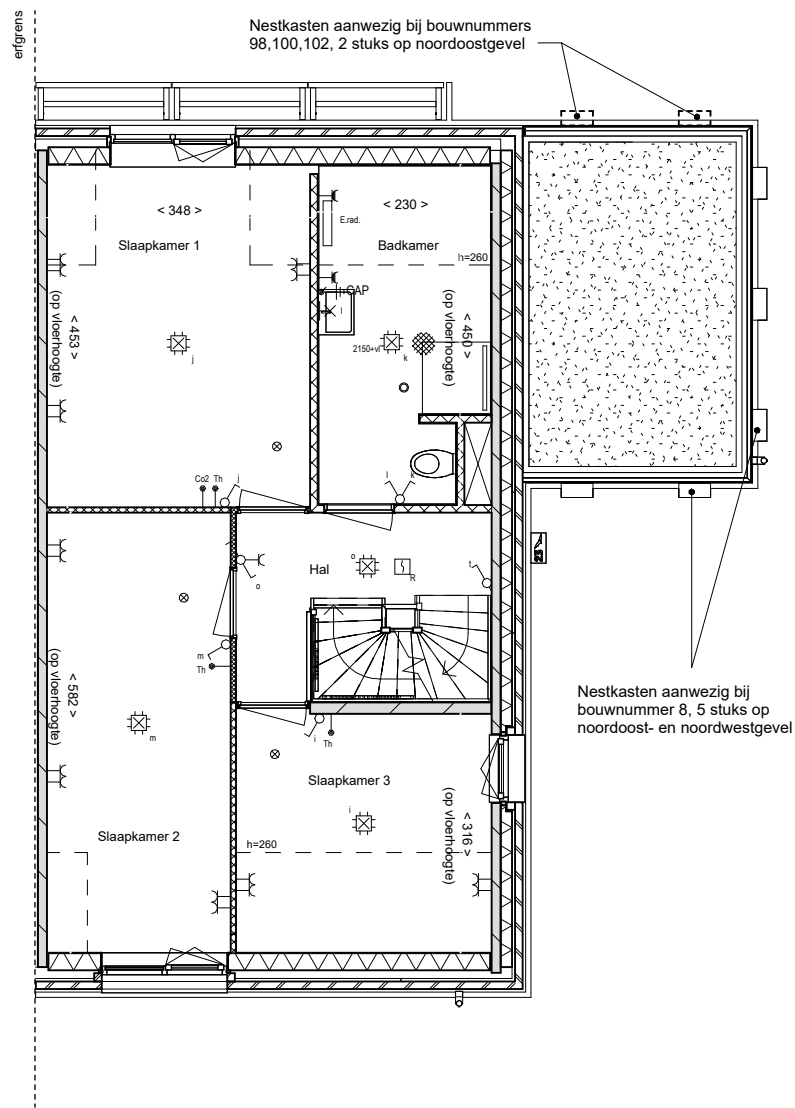
01 eerste verdieping
